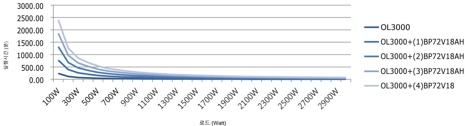
OL3000 실행시간 차트
