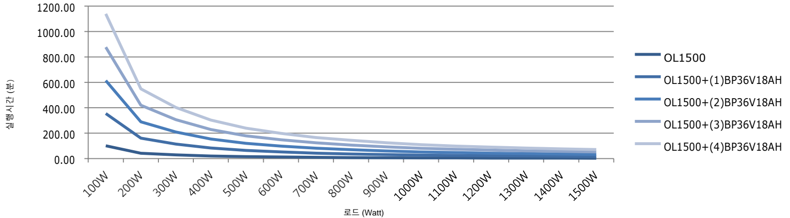
OL1500 실행시간 차트
