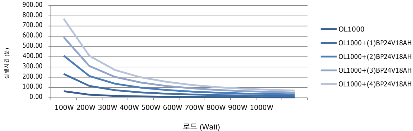
OL1000 실행 시간 차트
